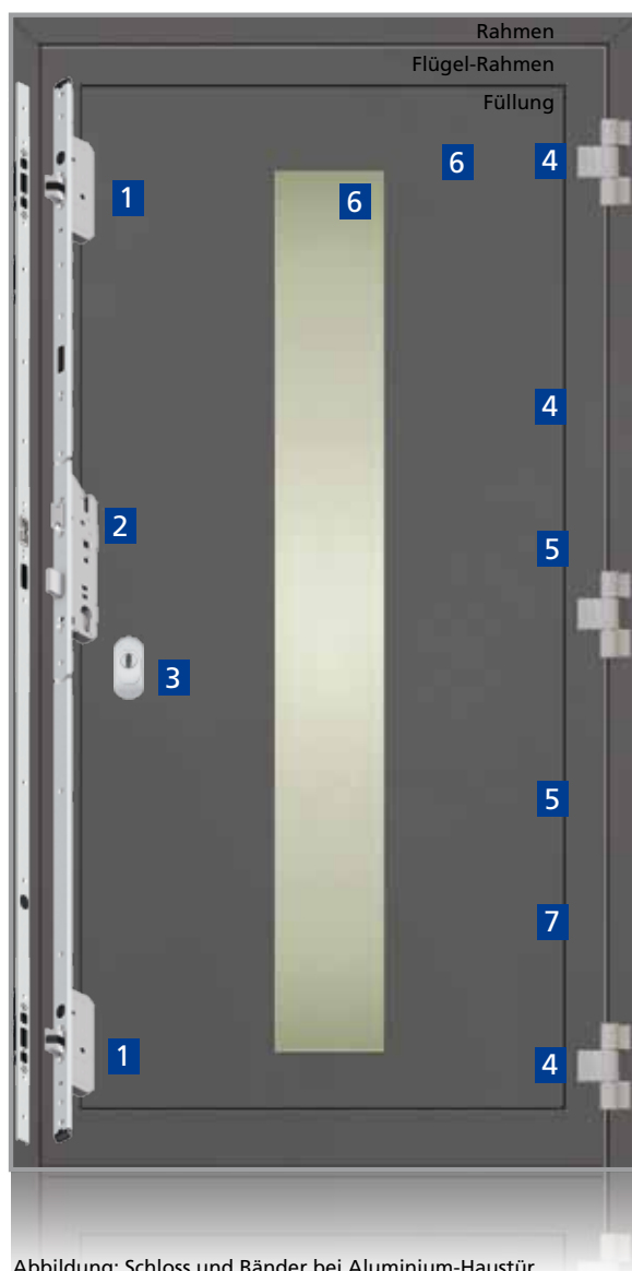
Abbildung: Schloss und Bänder bei Aluminium-Haustür
